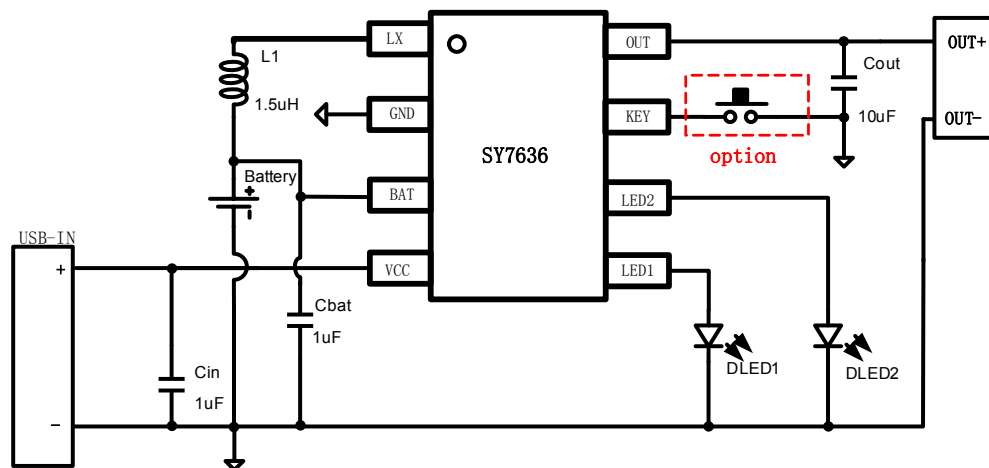
SY7636_KEY2L/SY7636_2L 应用电路
