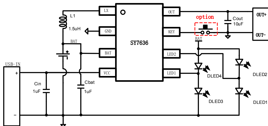
SY7636_KEY4L/SY7636_4L 应用电路
